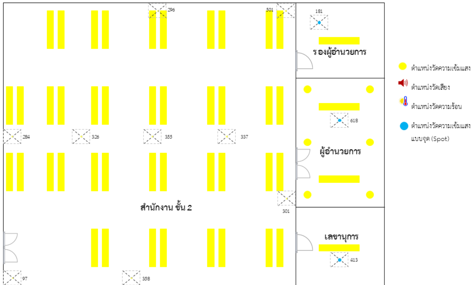
Lay out อาคารสำนักงานพิพิธภัณฑ์เรือนโบราณล้านนา สำนักส่งเสริมศิลปวัฒนธรรม ชั้น 2
